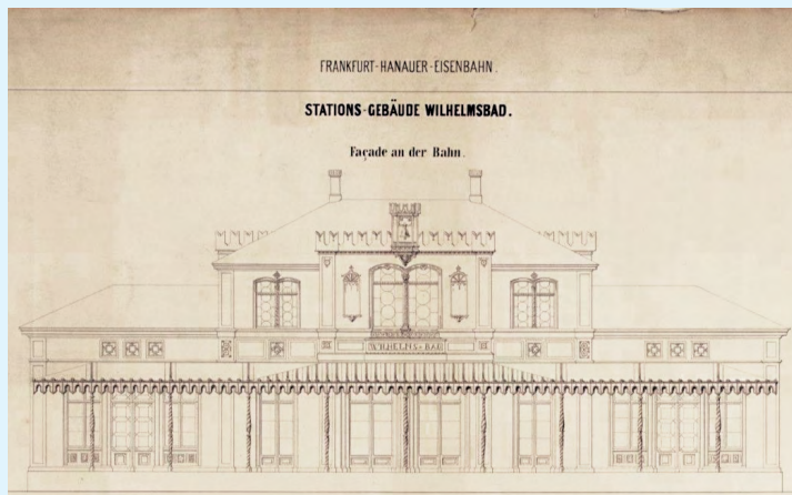
Entwurf des Bahnhofs Wilhelmshausen (Kassel) von 1846/47.
